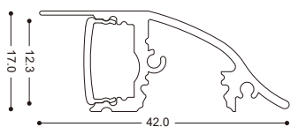
鋁材尺寸
