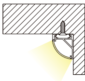
安裝說明
