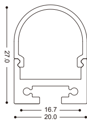
鋁材尺寸
