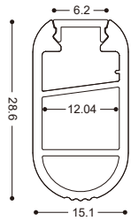
鋁材尺寸
