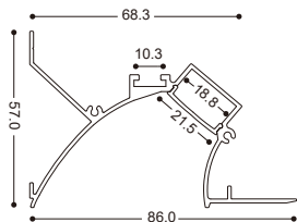
鋁材尺寸
