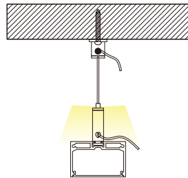
安裝說明
