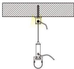
安裝說明
