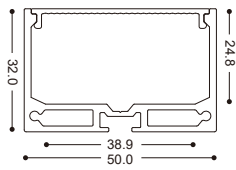
鋁材尺寸
