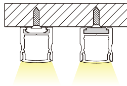
安裝說明
