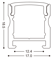
鋁材尺寸
