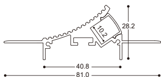
鋁材尺寸
