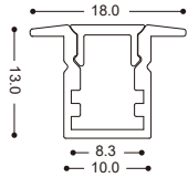
鋁材尺寸
