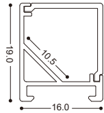
鋁材尺寸
