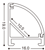
鋁材尺寸
