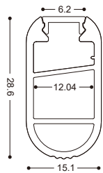
鋁材尺寸
