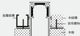
安裝示意
