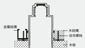
安裝示意
