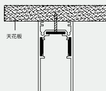
安裝示意
